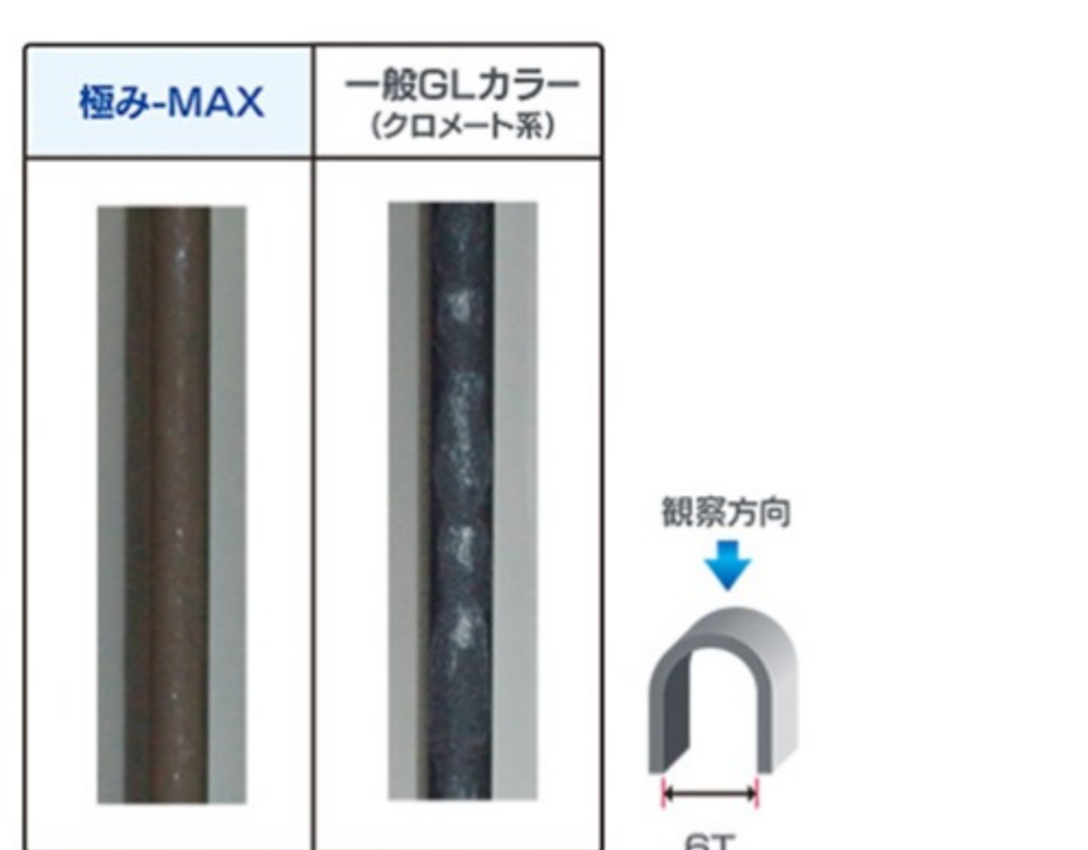
6T曲げ部 (CCT 150サイクル後の腐食状態)
