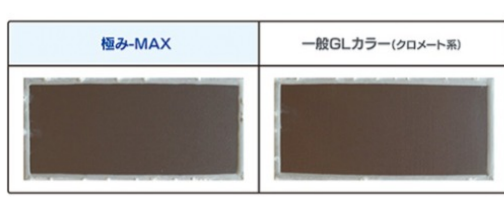
SST試験結果 (1500時間後試験片外観) 【平板 SST1500h後】
