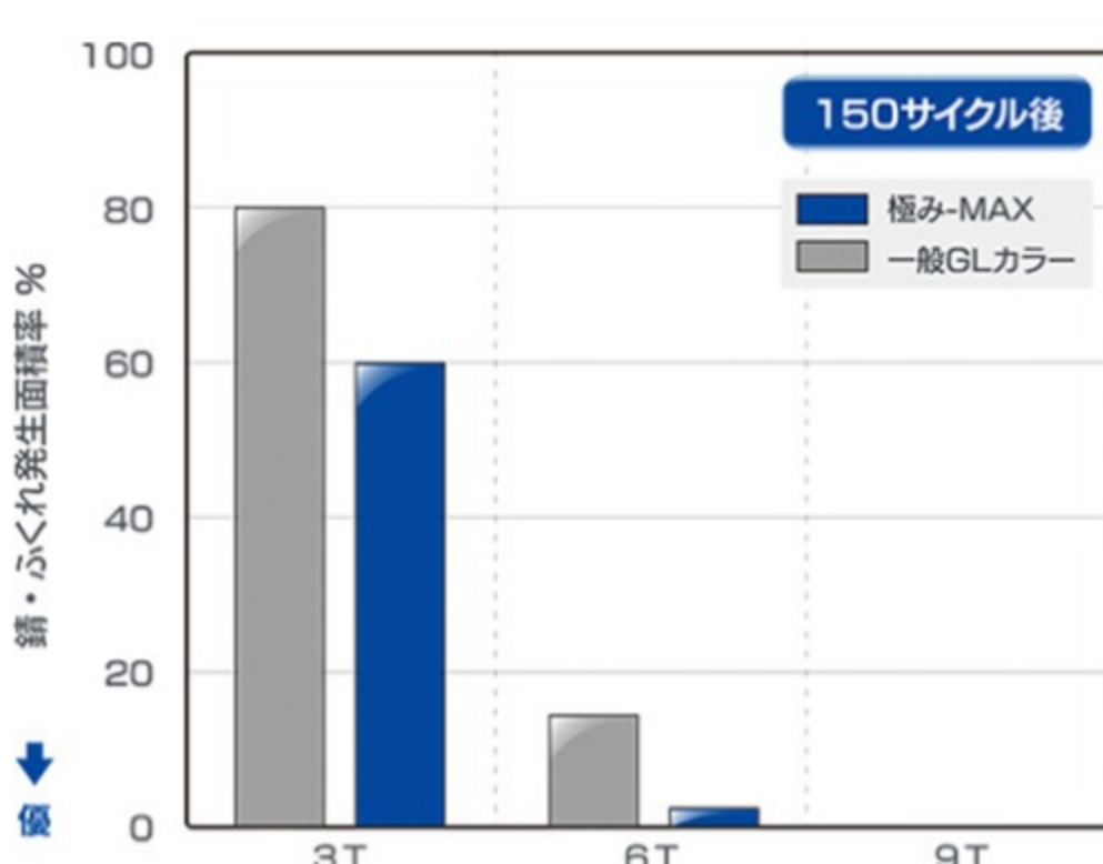
180度曲げ加工部の耐食性【複合サイクル腐食試験 150サイクル後の錆・膨れ発生面積率】
